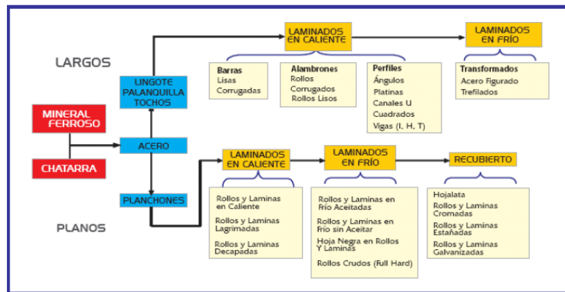
Figura 1. Diagrama proceso siderúrgico
