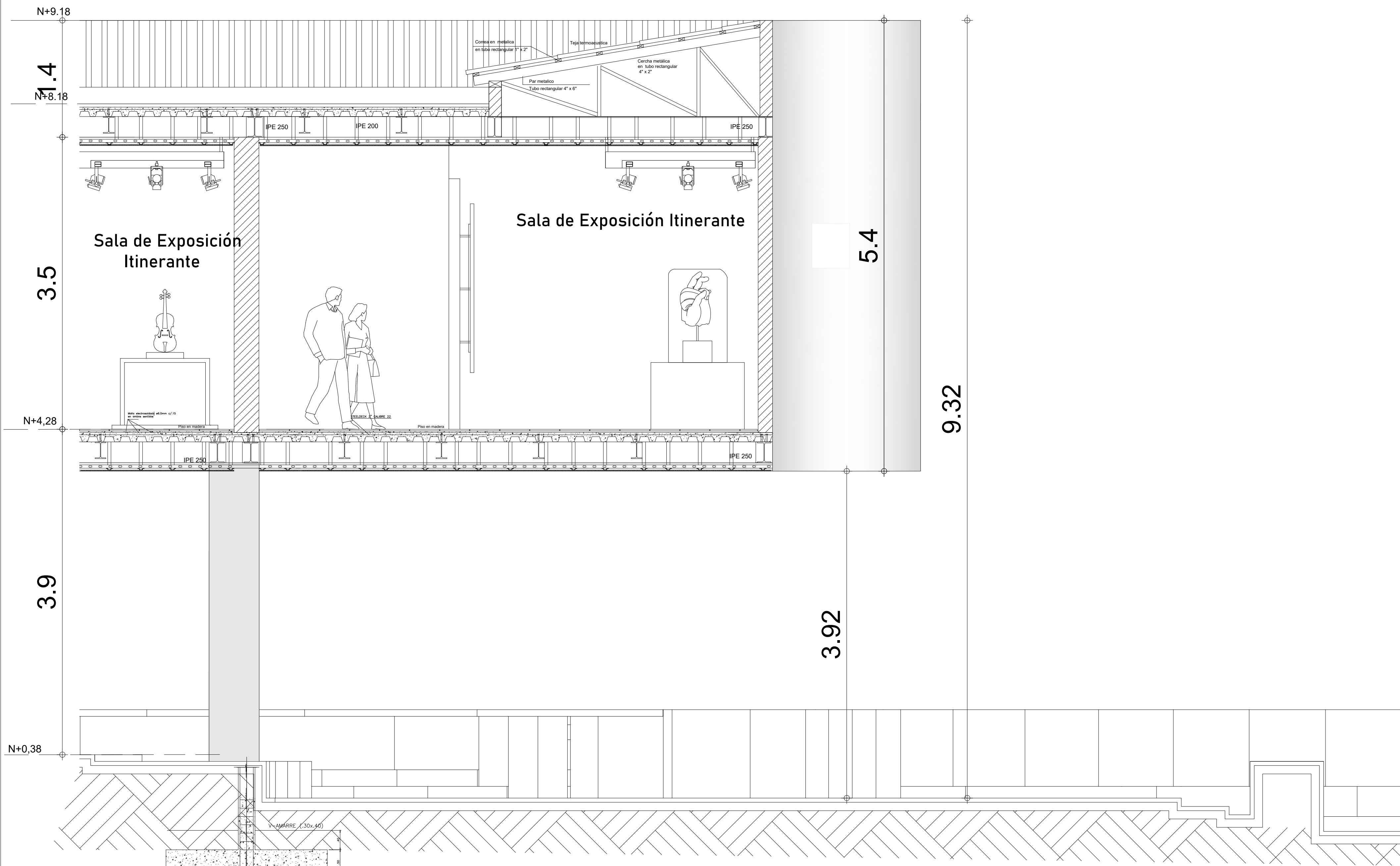
SECCIÓN A - A
