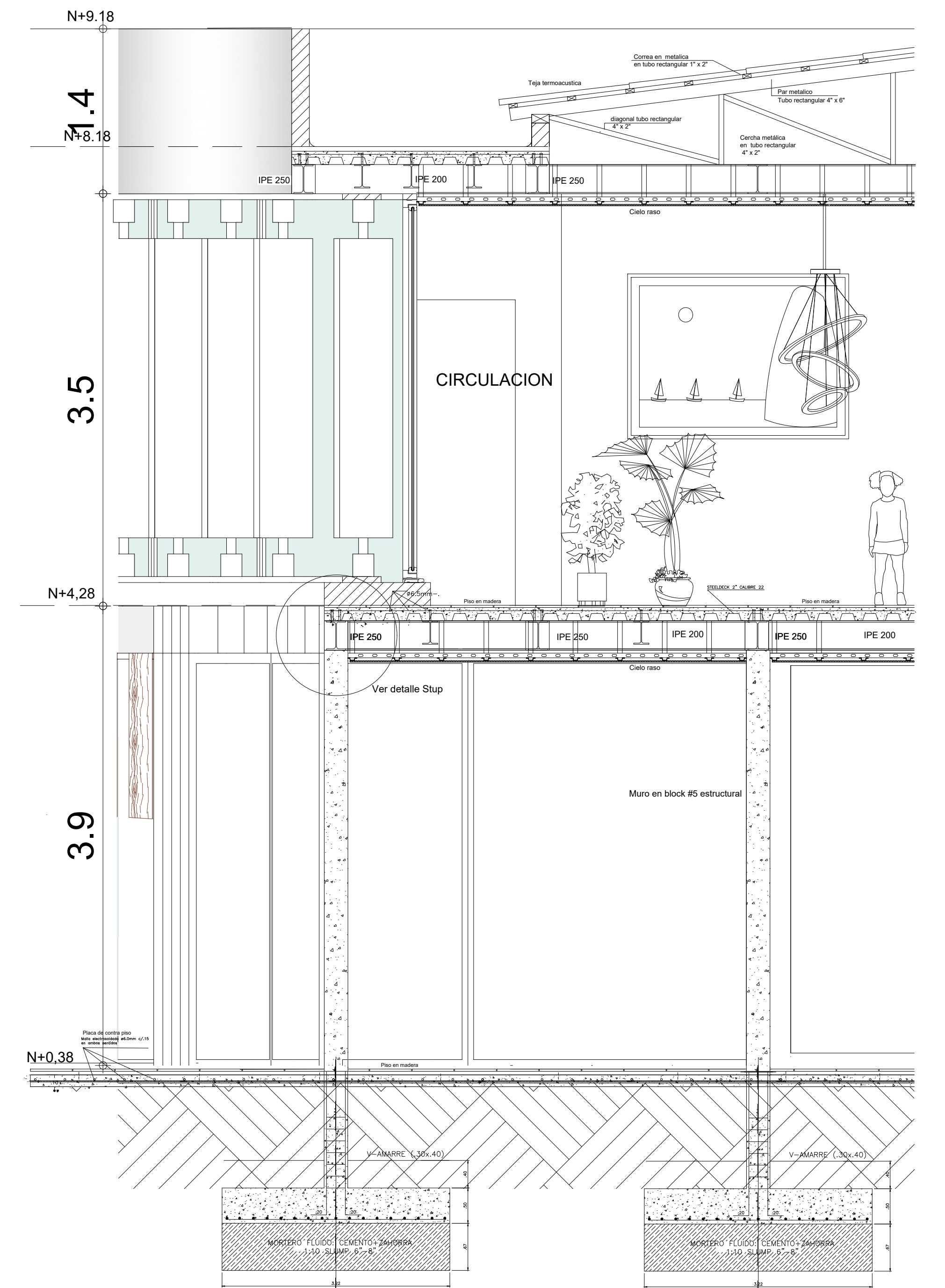
SECCIÓN C - C
