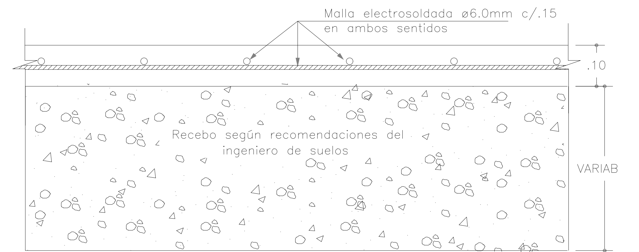
DETALLE PLACA DE CONTRA PISO
