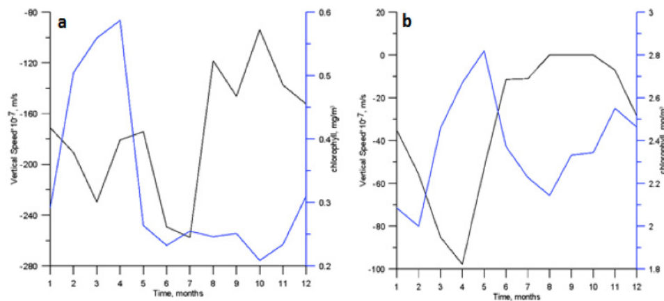
Figura 16. Oscilación anual de V_z y de clorofila a en el foco 3: 82°-83° W y 2° 30'-3° 30' N y en la zona costera: 6° 30' y 2° N
