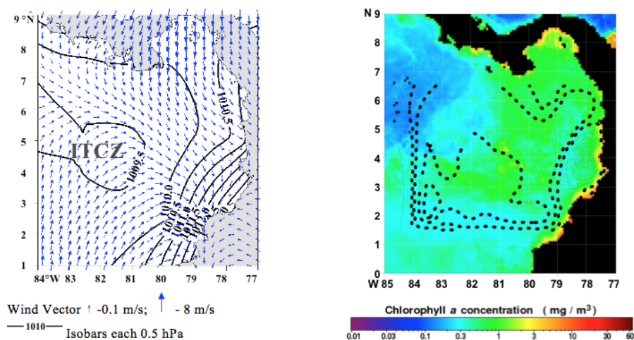
Figura 5. Campo de vientos, clorofila a (1997-2000) y zonas de surgencia (1971-2000) sobre la CPC en abril
