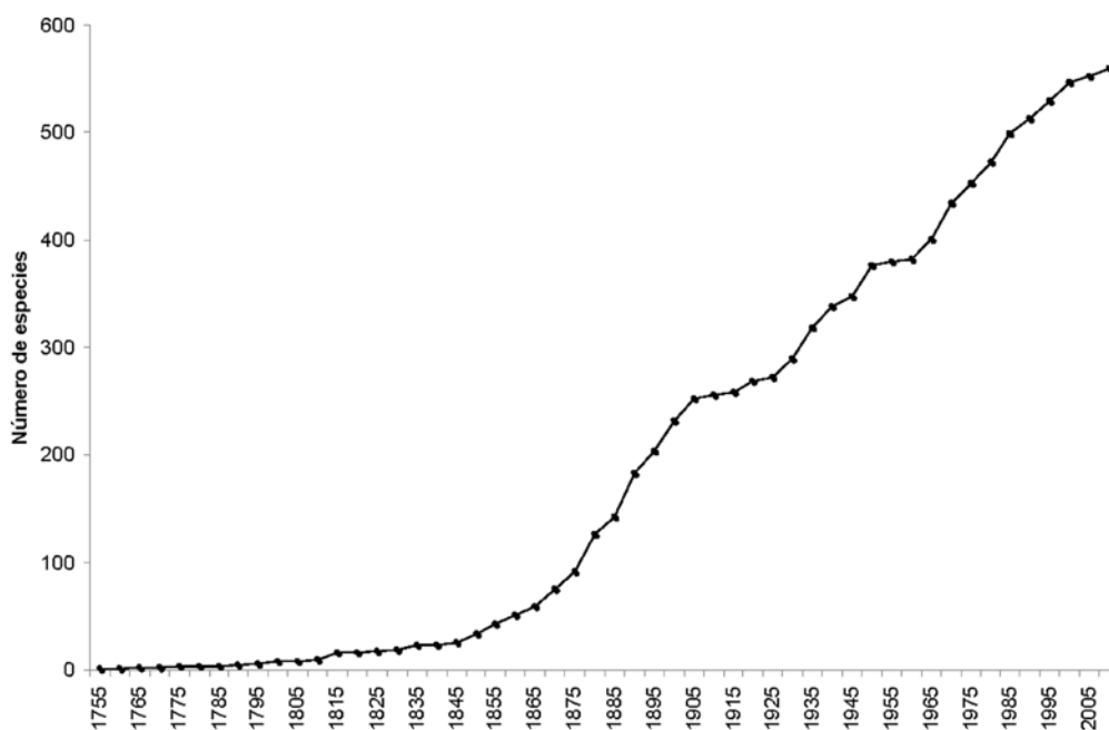
Figura 2. Curva acumulativa de descripción de especies de decápodos que se distribuyen en México, a partir de una muestra de 560 especies.
