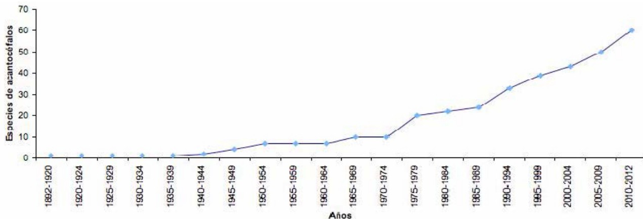
Figura 2. Curva acumulativa de especies de acantocéfalos por año de descripción (en intervalos de 5 años).
