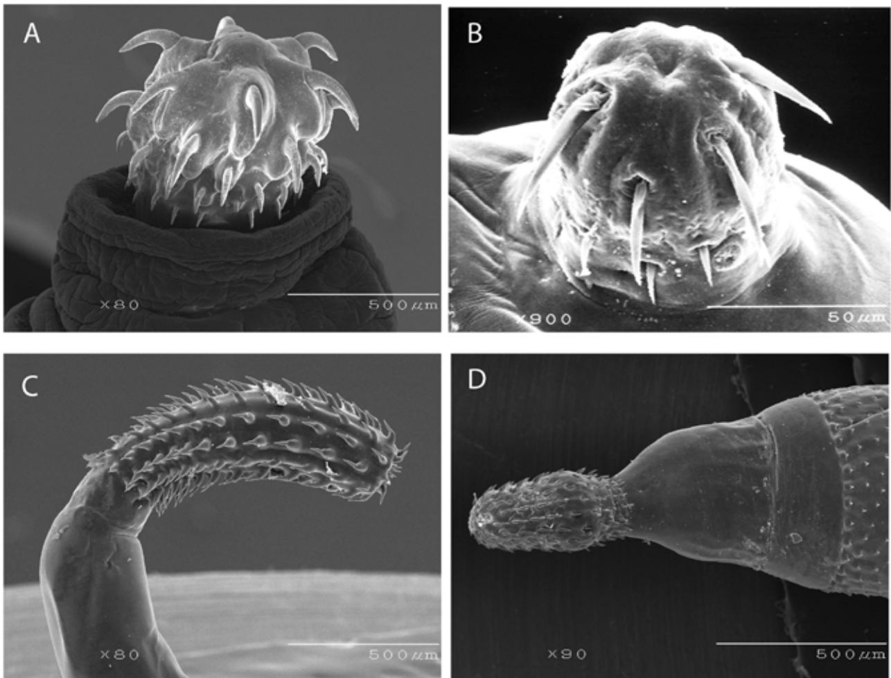
Figura 1. Representantes de la fauna mexicana de Acanthocephala. A, Oncicola sp.; B, Neoechinorhynchus brentnickoli Monks, Pulido-Flores y Violante-González, 2011; C, Aactorhynchus duranguensis Salgado-Maldonado, Aguilar-Aguilar y Cabañas-Carranza, 2005; D, Pseudocorynosoma anatarium (Van Cleave, 1945).
